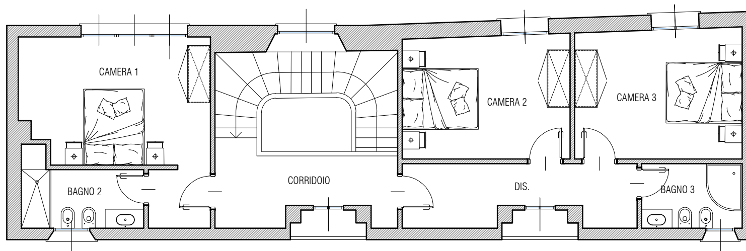
PIANO PRIMO
